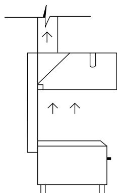
CORTE CAMPANA EXTRACCIÓN TIPO AMERICANA EN ANGULO
