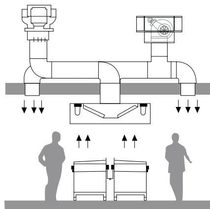
CORTE CAMPANA EXTRACCIÓN CON INYECCIÓN
