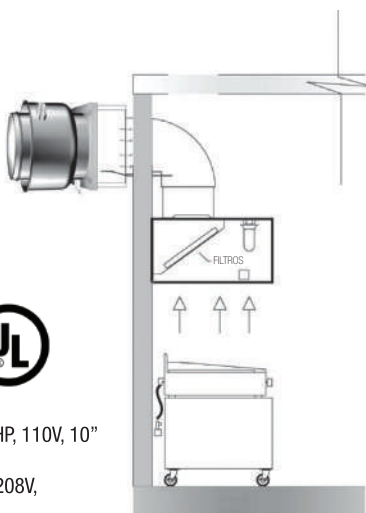
DETALLE DE EXTRACCIÓN A LA PARED
