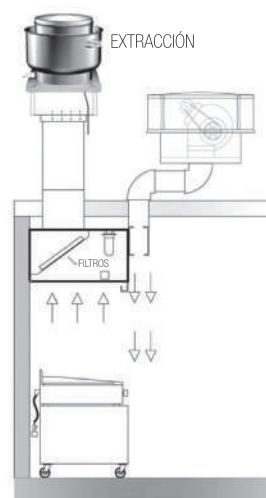
DETALLE DE EXTRACCIÓN AL TECHO CON INYECTOR
